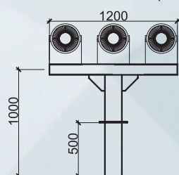
Držák K1-1.2-1.0 (M1ак, M2ак)
