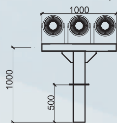
Držák K1-1.0-1.0 (M1ак, M2ак)
