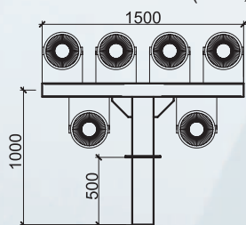
Držák K1-1.2-1.0 (M1ак, M2ак)
