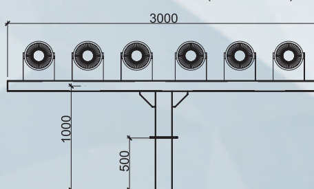
Držák K1-3.0-1.0 (M1ак, M2ак)
