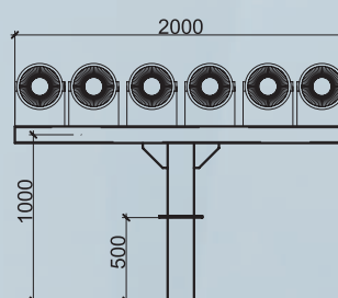
Držák K1-2.0-1.0 (M1ак, M2ак)
